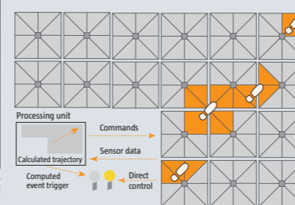
Abb. 2: SensFloor Underlay mit dreieckigen Sensorflächen. Schritte erzeugen Sensorsignale, die zu einem Empfänger gefunkt und dort ausgewertet werden.
